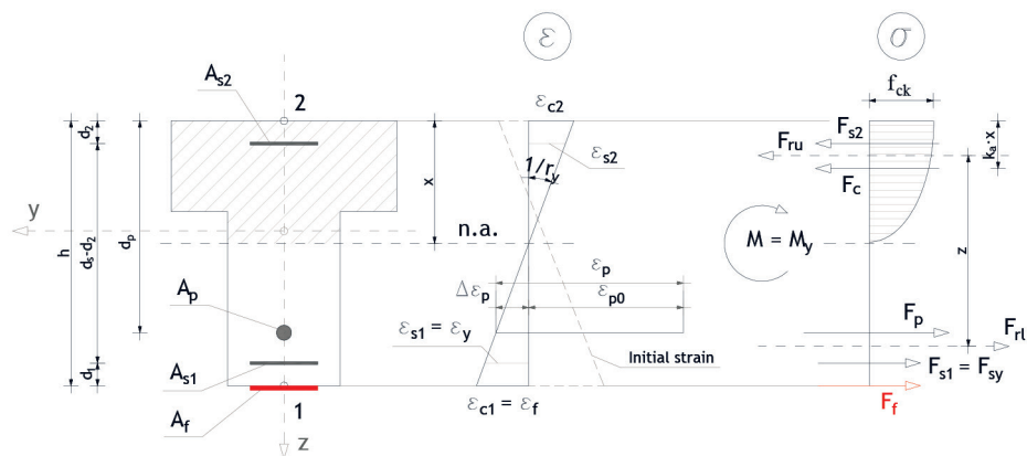
Slika 3. Raspodjela relativnih deformacija i naprezanja u poprečnom presjeku pojačane prednapete AB grede u trenutku popuštanja armature
