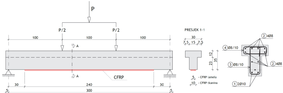
Slika 5. Geometrijske karakteristike analizirane prednapete AB grede
