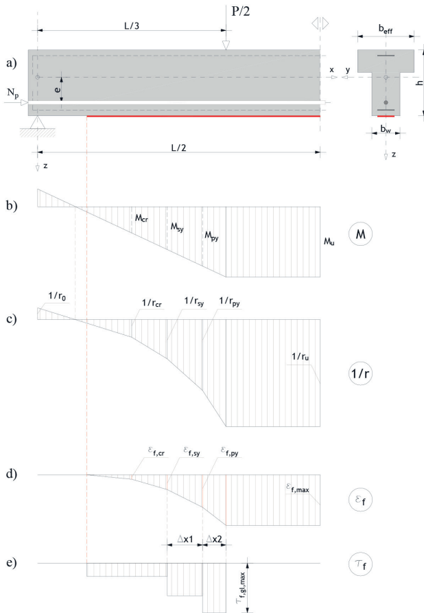
Slika 4. Prikaz prednapete AB grede; te dijagrama momenta savijanja ( M ), zakrivljenosti ( 1/r ), relativne deformacije FRP lamele ( \varepsilon_f ) i naprezanja prijanjanja ( \tau_f )
